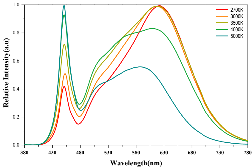
CRI(Ra) 90Min
